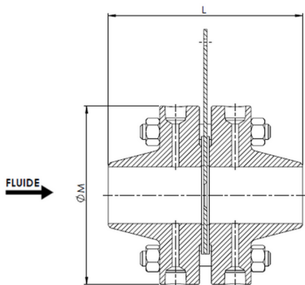
Débitmètre 25/25 RF
