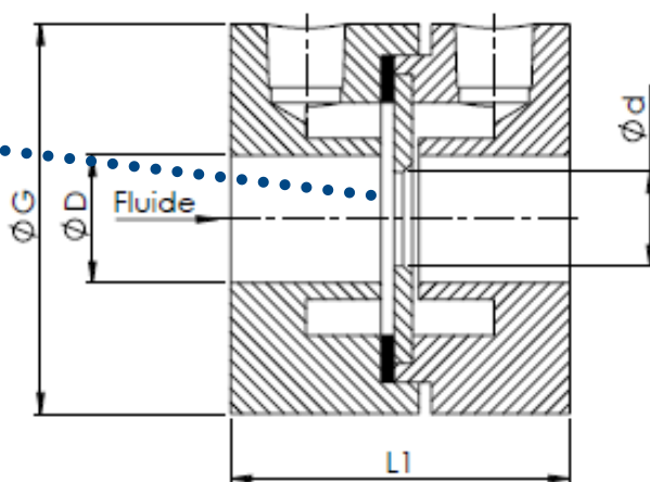
Débitmètre o/o avec chambre annulaire
