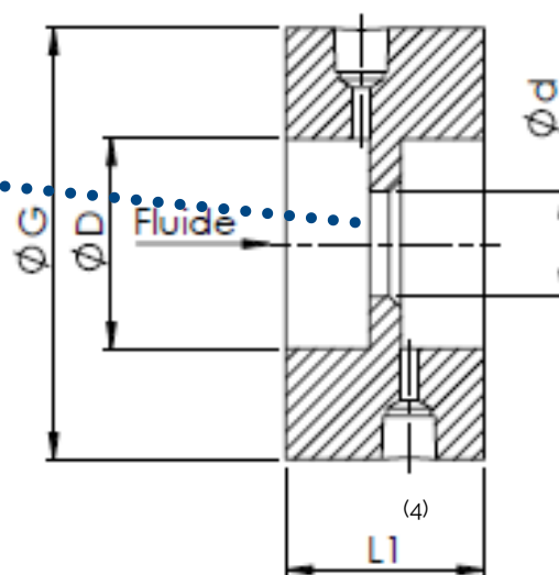
Débitmètre 0/0 avec monobloc
