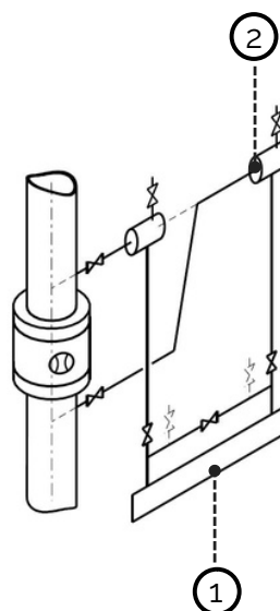
Fig 4 : Montage transmetteur avec pots de condensation sur canalisation verticale
