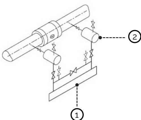
Fig 3 : Montage transmetteur avec pots de condensation sur une canalisation horizontale
