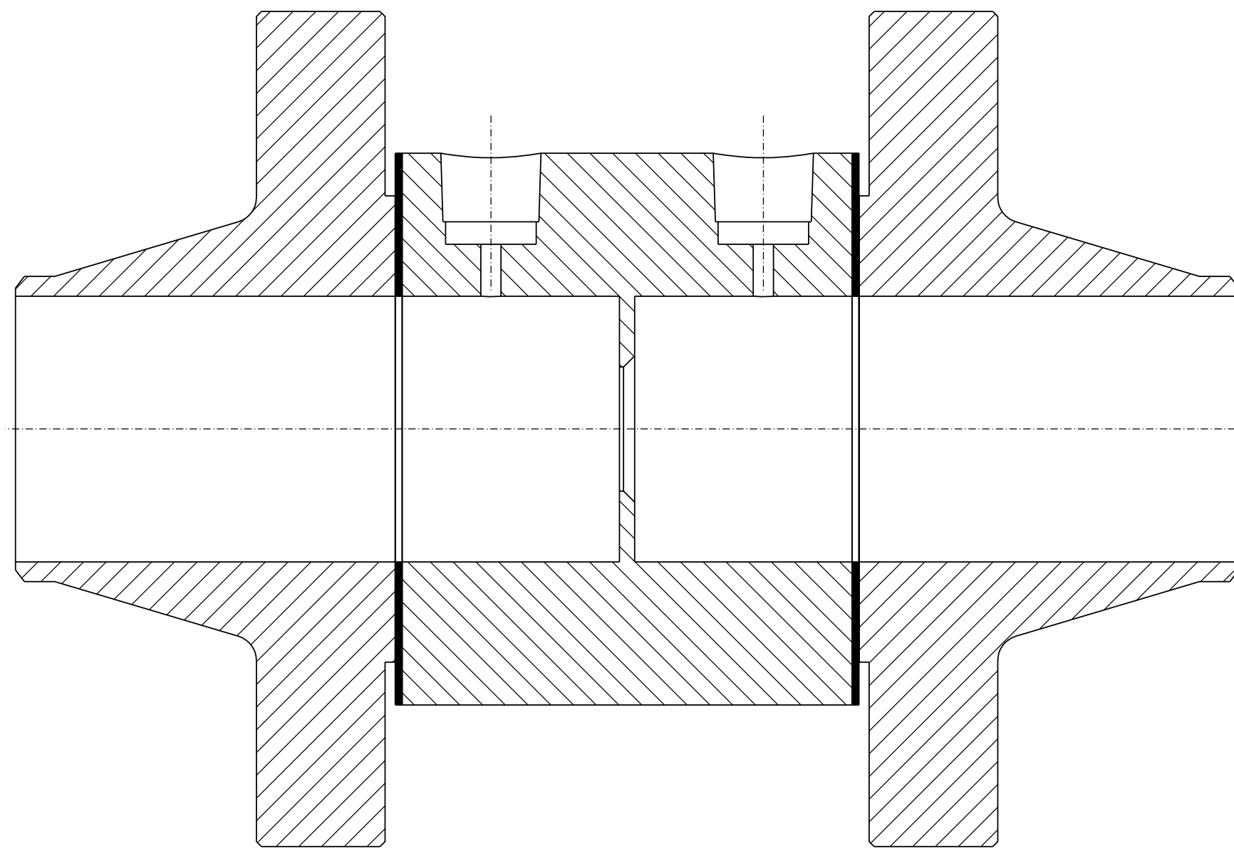
COUPE D-D ECHELLE 1:1
