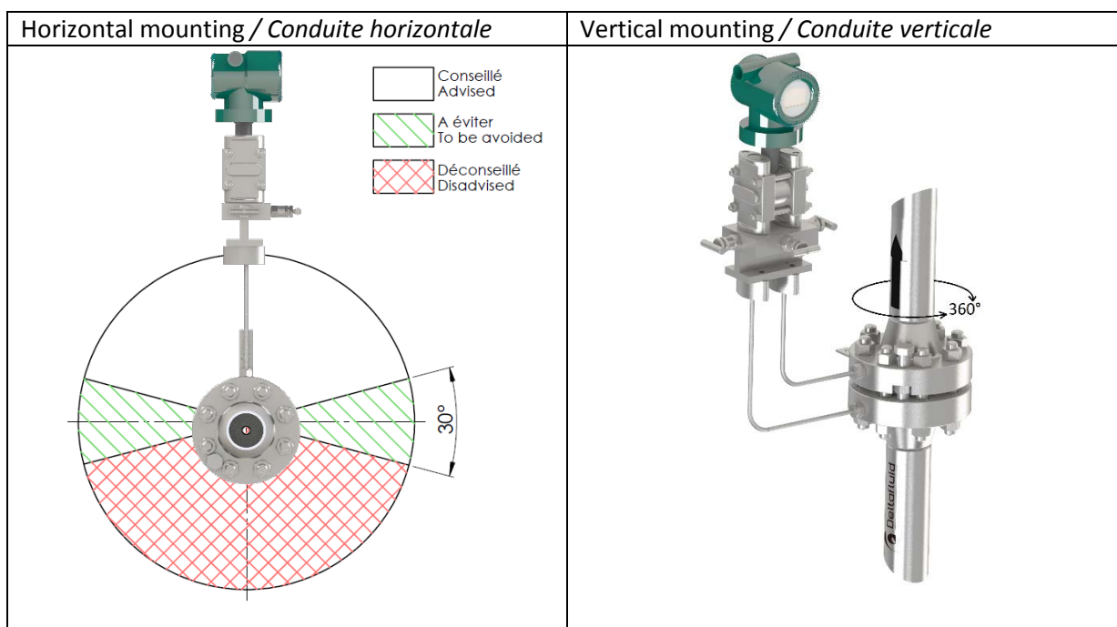
Fig 6 : Transmitter mounting for gas applications Fig 6 : Montage du transmetteur pour une application avec un fluide gazeux
