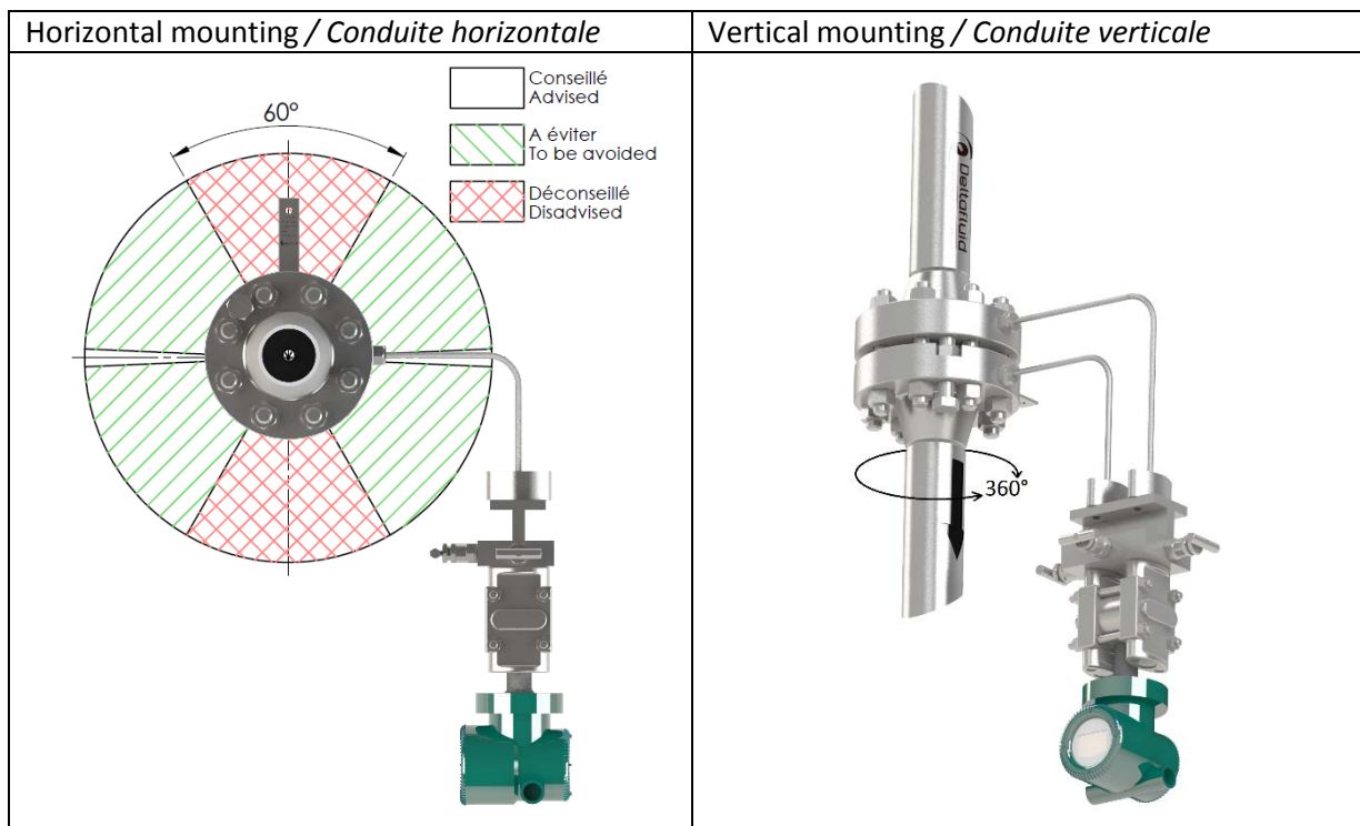
Fig 7 : Transmitter mounting for steam applications Fig 7 : Montage du transmetteur pour une application avec de la vapeur
