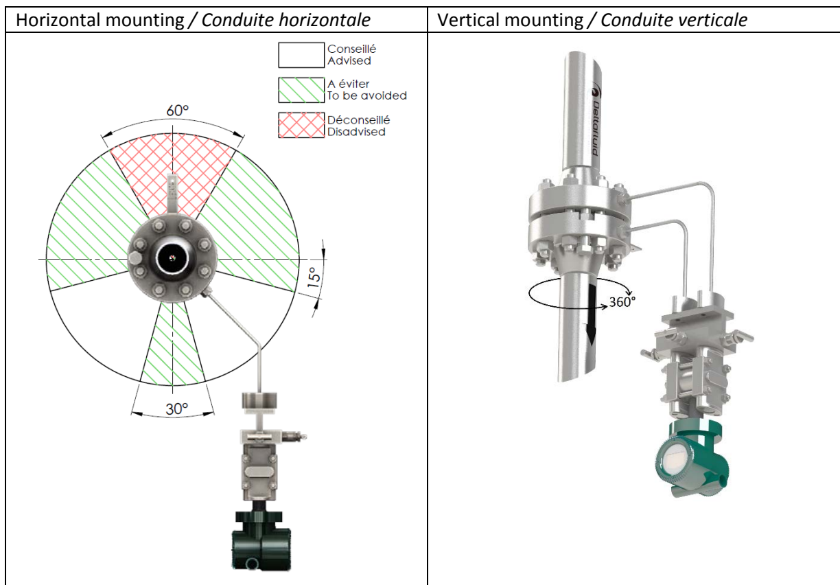
Fig 5 : Transmitter mounting for liquid applications Fig 5 : Montage du transmetteur pour une application avec un fluide liquide
